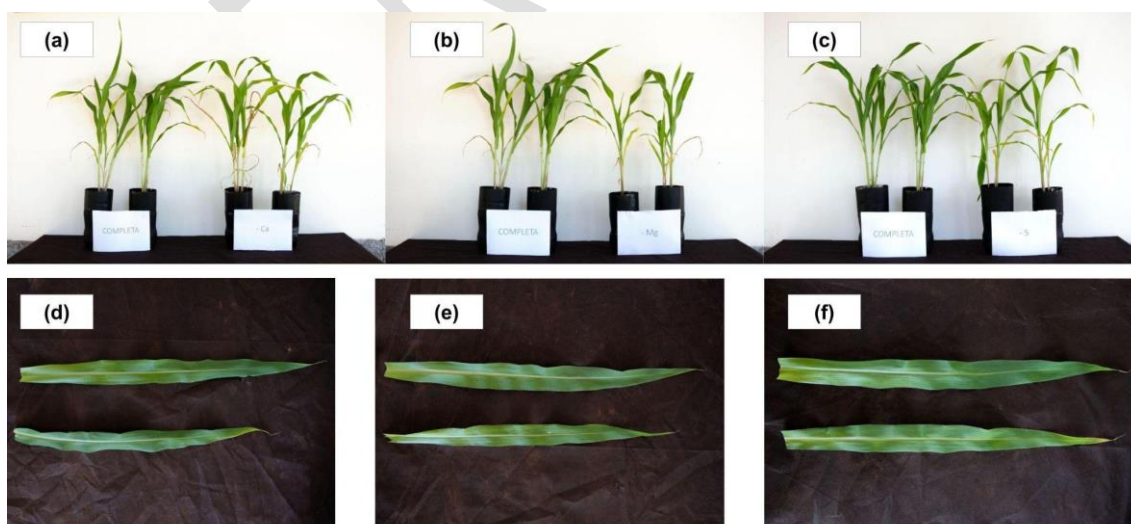
Figura 1: Sintomas visuais da deficiência de Ca (a) e (d), Mg (b) e (e) e S (c) e (f) em plantas de sorgo cultivadas em solução nutritiva.
