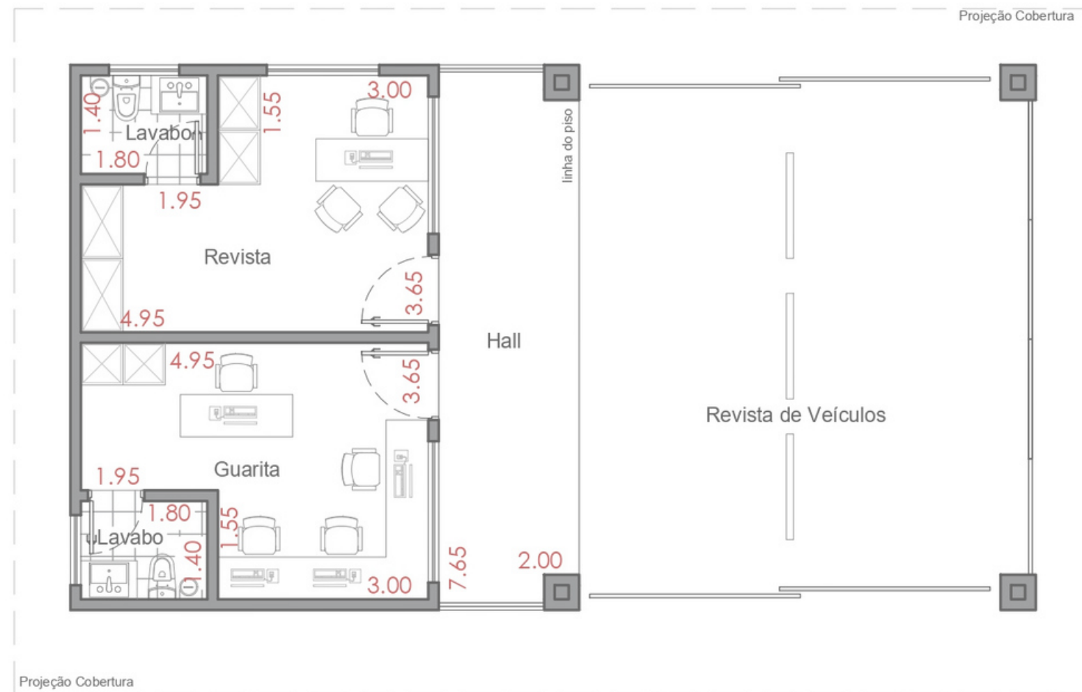
Figura 38 - Planta Layout - Acesso e controle.
