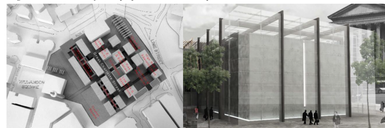
Figura 15 e 16 – Locação do projeto no terreno e Capela ecumênica.
