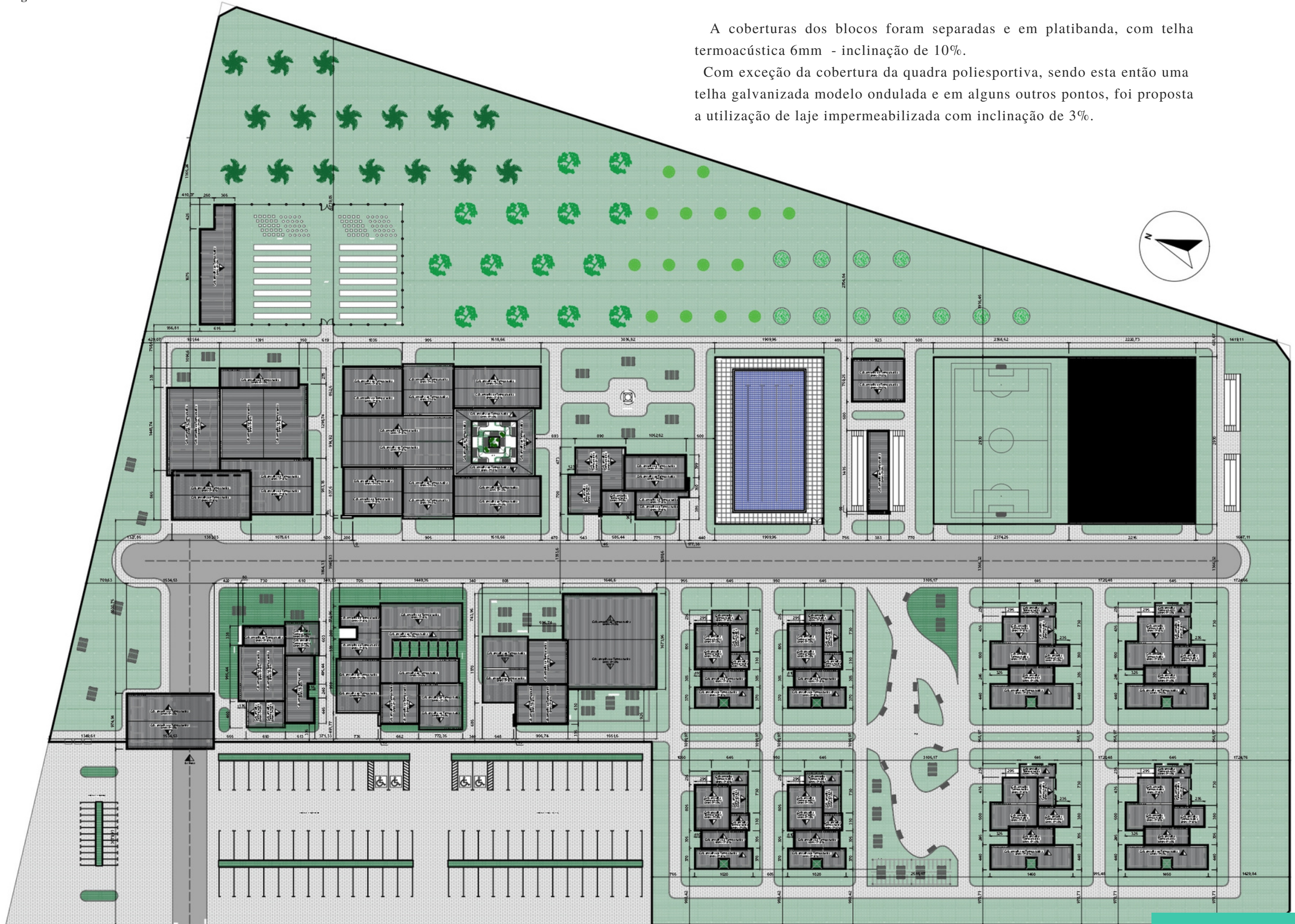
Figura 36 - Planta cobertura.
