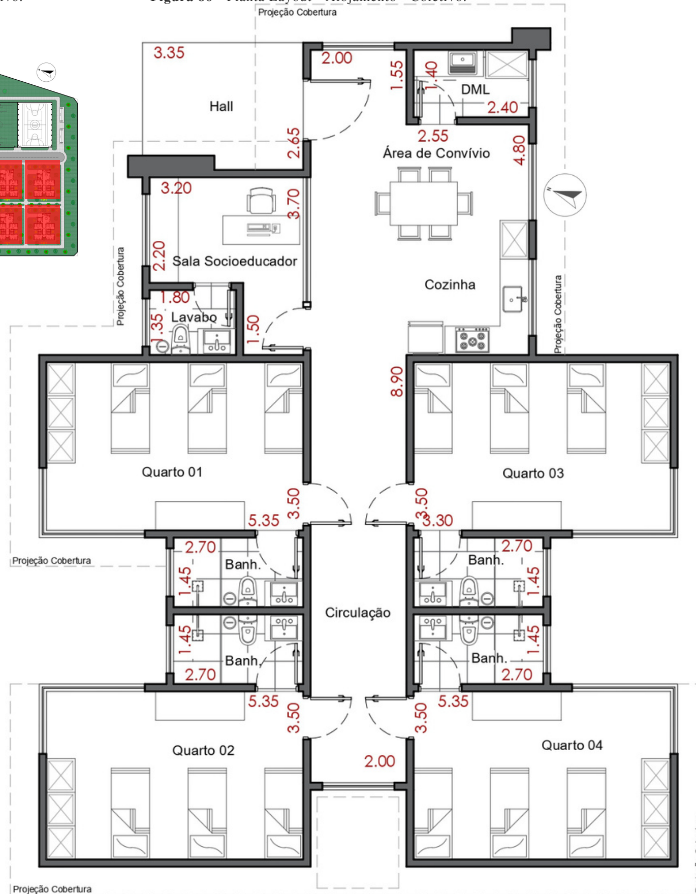
Figura 86 - Planta Layout - Alojamento - Coletivo.
