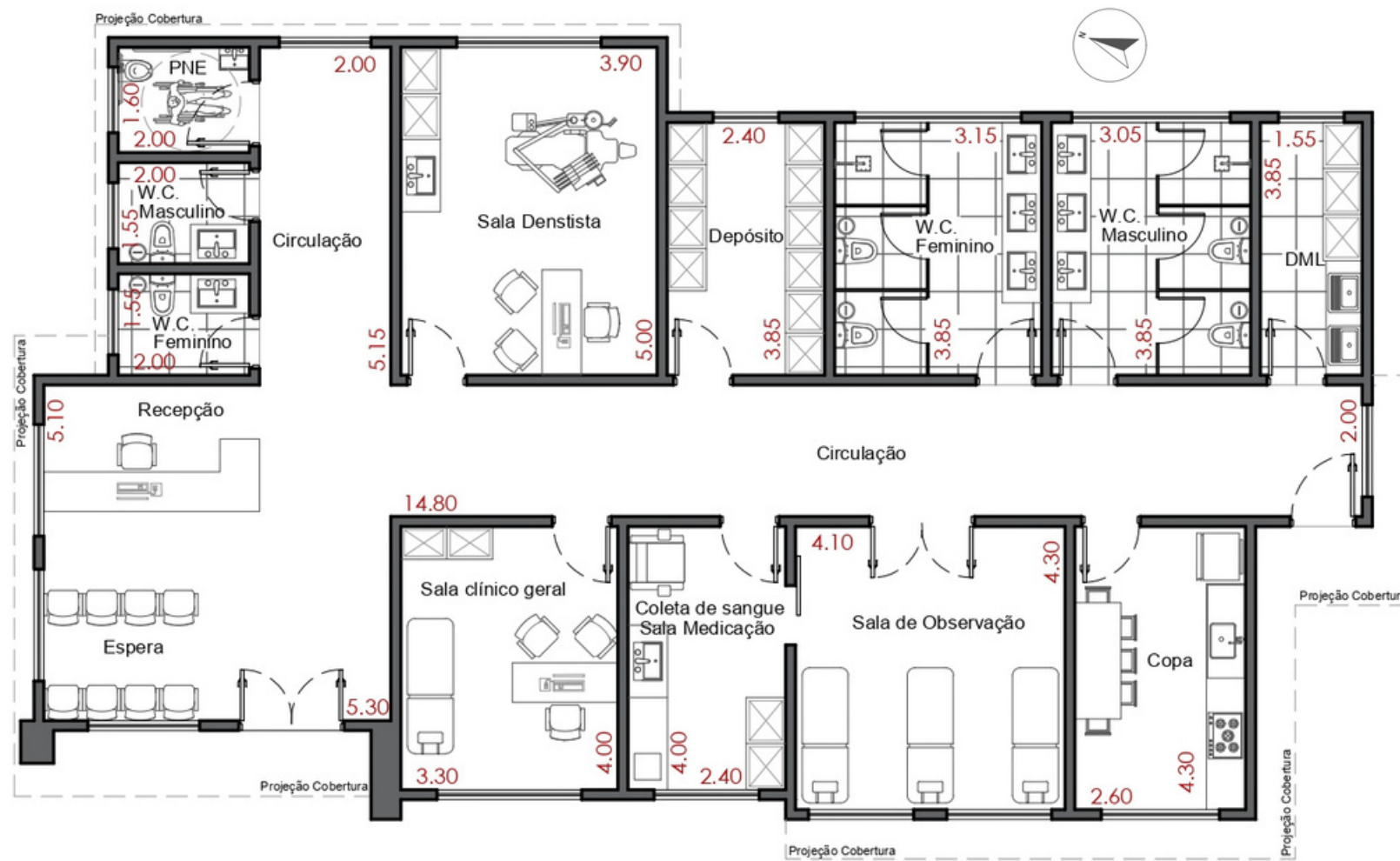
Figura 74 - Planta Layout - Serviço e refeitório.
